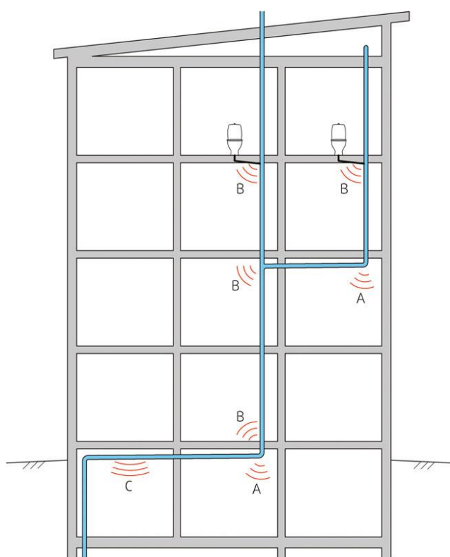
Fig. 5 Typiske monterings-situasjoner for avløpsrør. Orienterende verdier for referansesituasjonene A–C er gitt i tabell 3. Fra Byggforskserien 553.182 Støy fra avløpsinstallasjoner .
