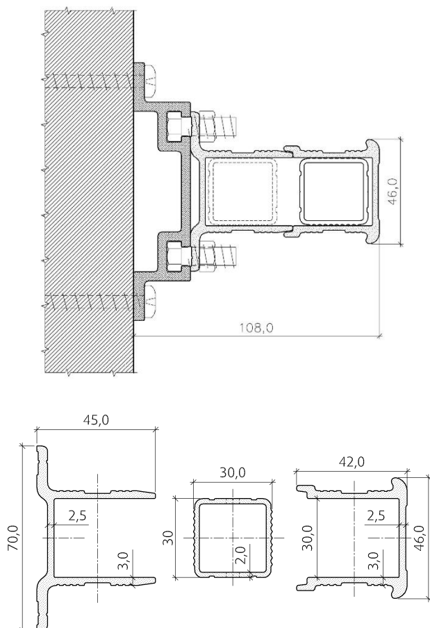
Fig. 3 Snitt av sammenslått stige og profiler til indre vange, trinn og ytre vange.
