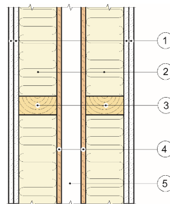
Horizontalsnitt
