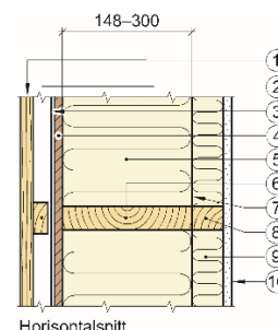
Horizontalsnitt
