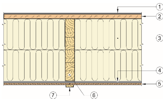
Vertikalsnitt
