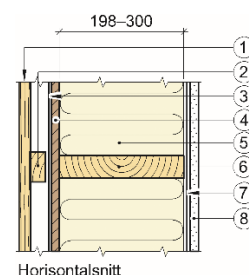
Horizontalsnitt
