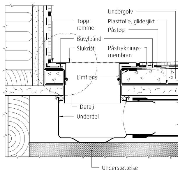
Fig. 3 Blücher designsluk plassert mot en vegg med undertøttelse. Butylbåndet i overgang golv/vegg må være minst 100 mm bredt og dekke hele limflensen. Mot veggens skal butylbåndet trekkes opp langs veggens.
