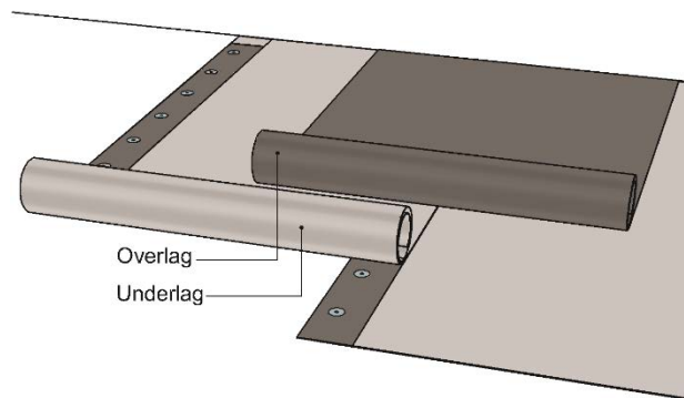
Fig. 1 Katepal 2-lag extra asfalt takbelegg består av en overlagstekning som helsveises til et mekanisk festet underlagsbelegg.
