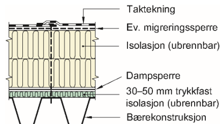
Fig. 2 BMI Dampsperre monteret i kompakt takkonstruksjon
