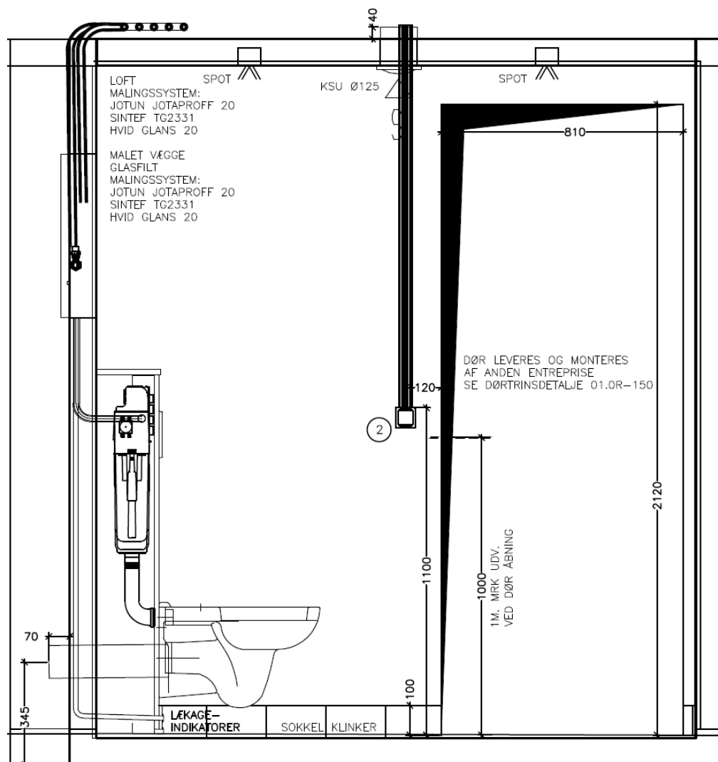
Fig. 2 Vertikalsnitt viser oppbygging av gulv, vegger og tak samt fordelerskap i vegg og innkasset systerne Figur: Ready Bathroom ApS
