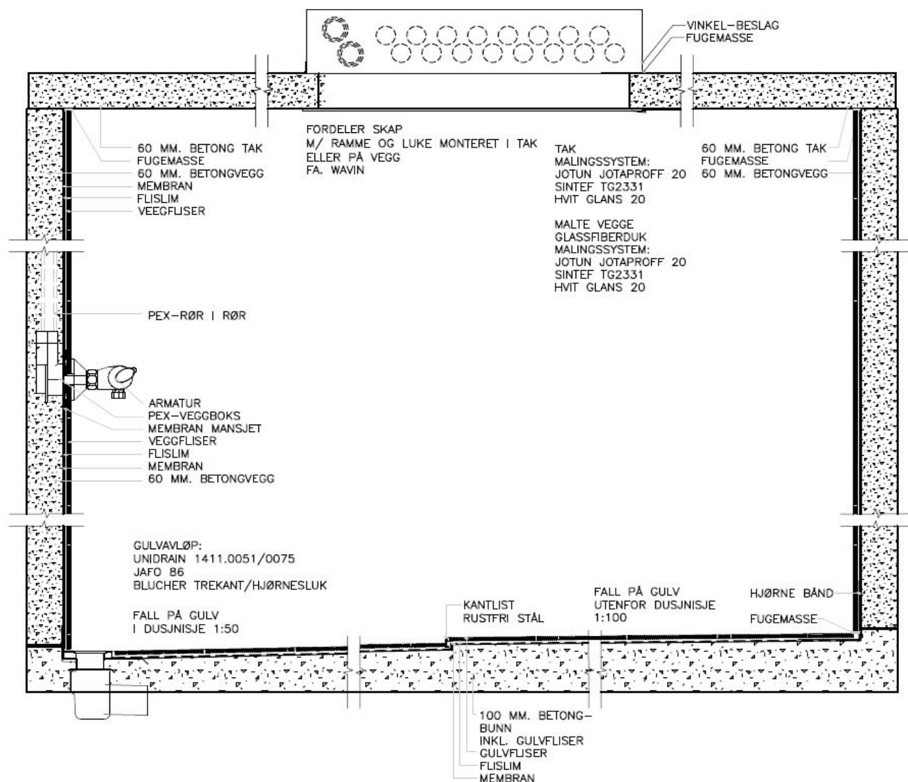
Fig. 2 Vertikalsnitt
