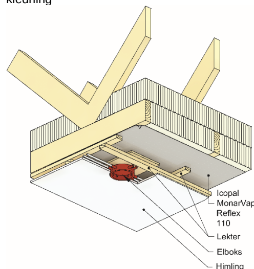
Fig. 2 Tak med lukket luftrom mellom MonarVap® Reflex 110 reflekterende dampspærre og himling.
