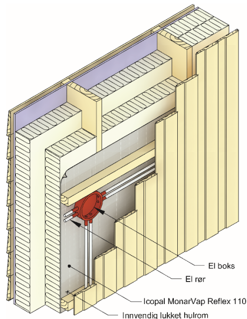
Fig. 1 Bindingsverksvegg med lukket luftrom mellom MonarVap® Reflex 110 reflekterende dampspærre og innvendig kledning
